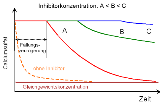
Kristallisationsverlauf in Gegenwart von Fällungsverzögerern
