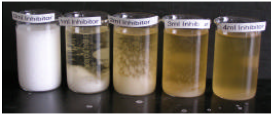
Gipsfällung in Abhängigkeit von der Inhibitorkonzentration
