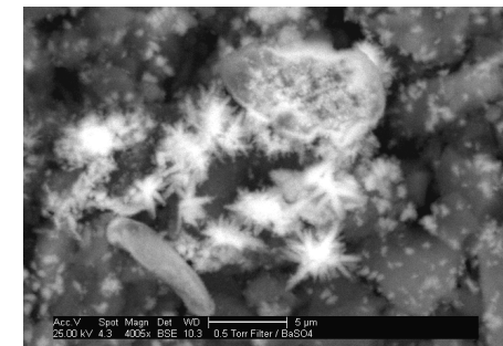
In einem porösen Sandstein gebildete \text{BaSO}_4 -Kristalle
